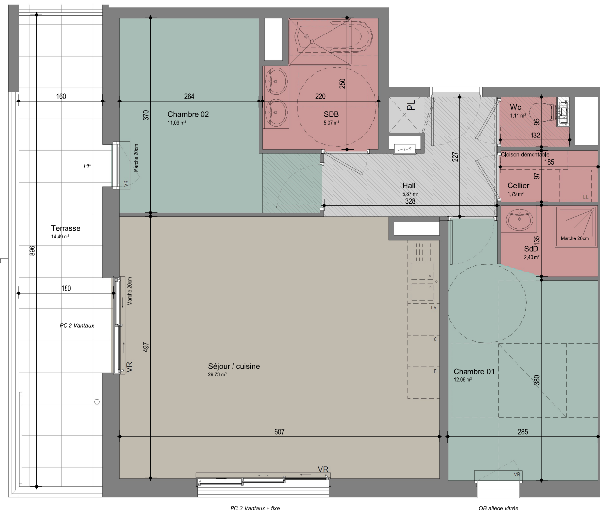
PC 3 Vantaux + fixe
